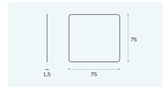
IN.26.2 Pictogramas aplicados em aço inox de 1,5mm para aplicação paralela à parede. Com fixação por adesivo extra-forte / Stainless steel pictograms with 1,5mm thickness for application parallel to the wall. With strong adhesive fixing / Sinalética en acero inox de 1,5mm para uso paralelo a la pared. Con sujeción por adesivo extra-fuerte.
